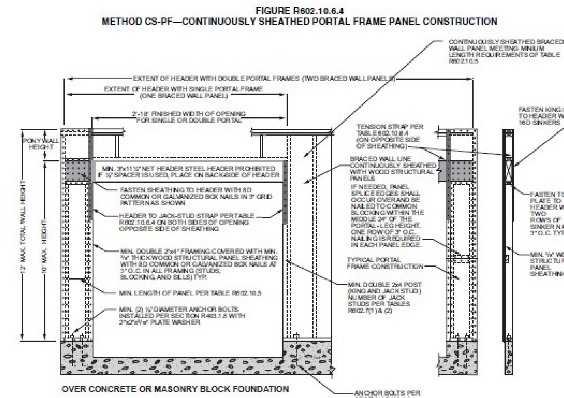
7 R602.10.6.4 CS-PF METHOD NOT TO SCALE
